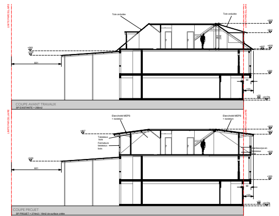
COUPES EXISTANT / PROJET
