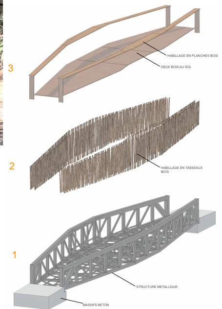
SCHEMA MONTRANT LA STRUCTURE METALLIQUE ET L'HABILLAGE BOIS
