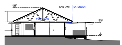
COUPE PROJET
