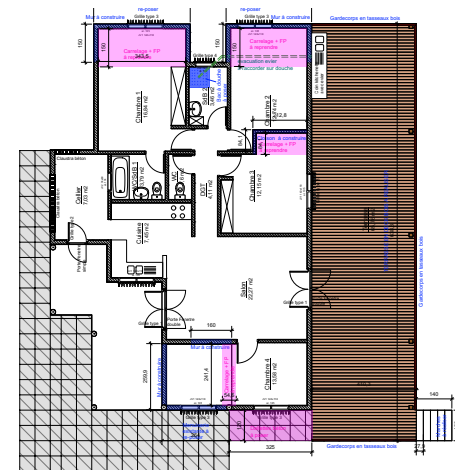
PLAN PROJET
