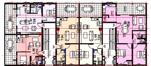
PLAN ETAGE COURANT
